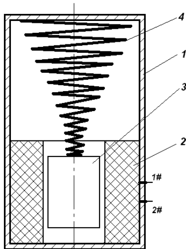
Рисунок 4. Конструкція сеймосенсора
