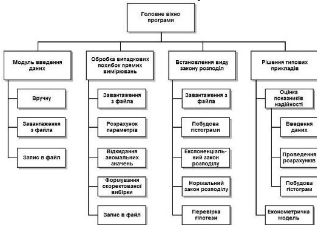
Рисунок 1. Структурна схема розробленого програмного забезпечення
